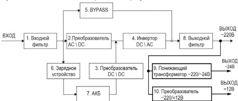
Рисунок 4 - функциональная схема изделия
